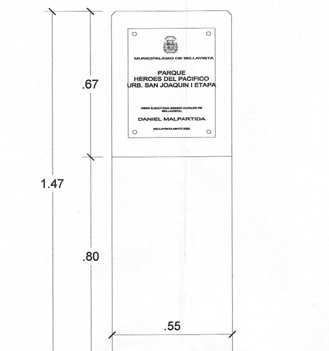
ELEVACION FRONTAL
