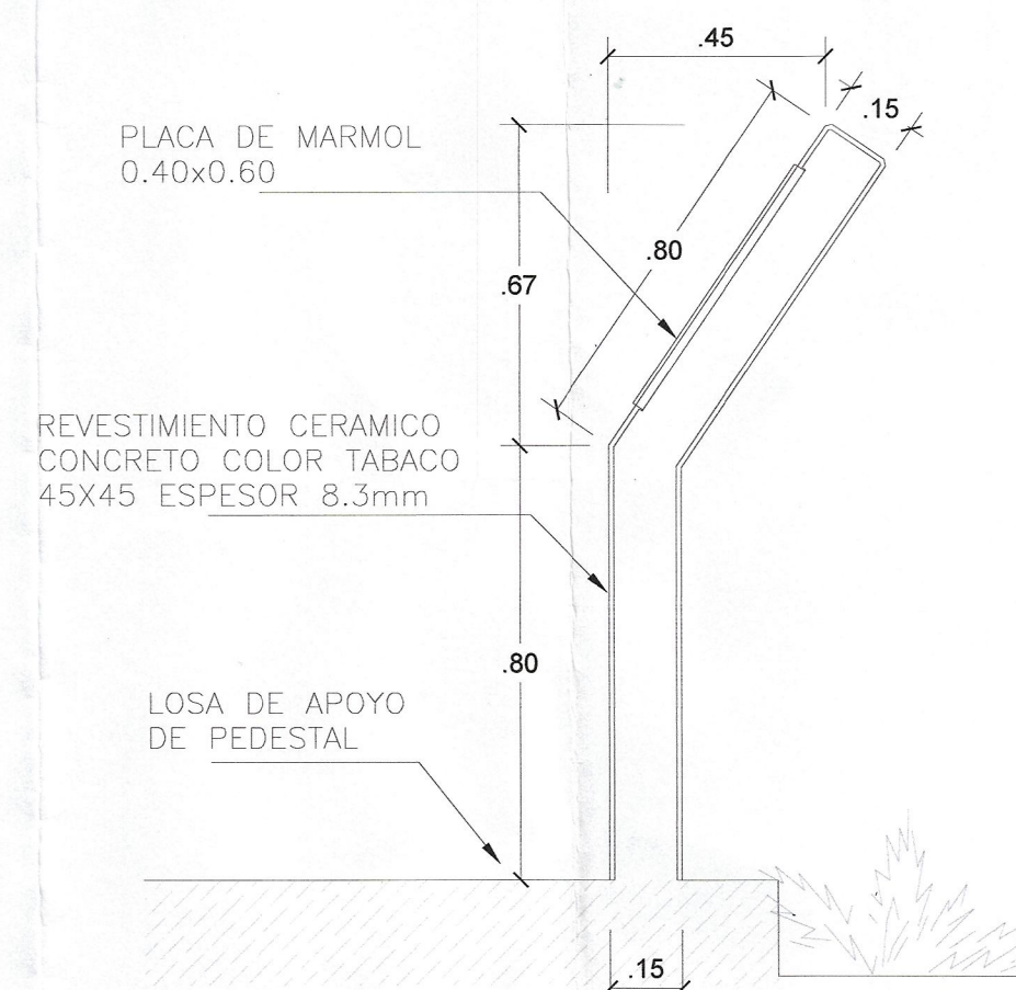
CORTE 1-1
