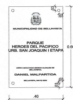
DETALLE DE PLACA DE MARMOL
