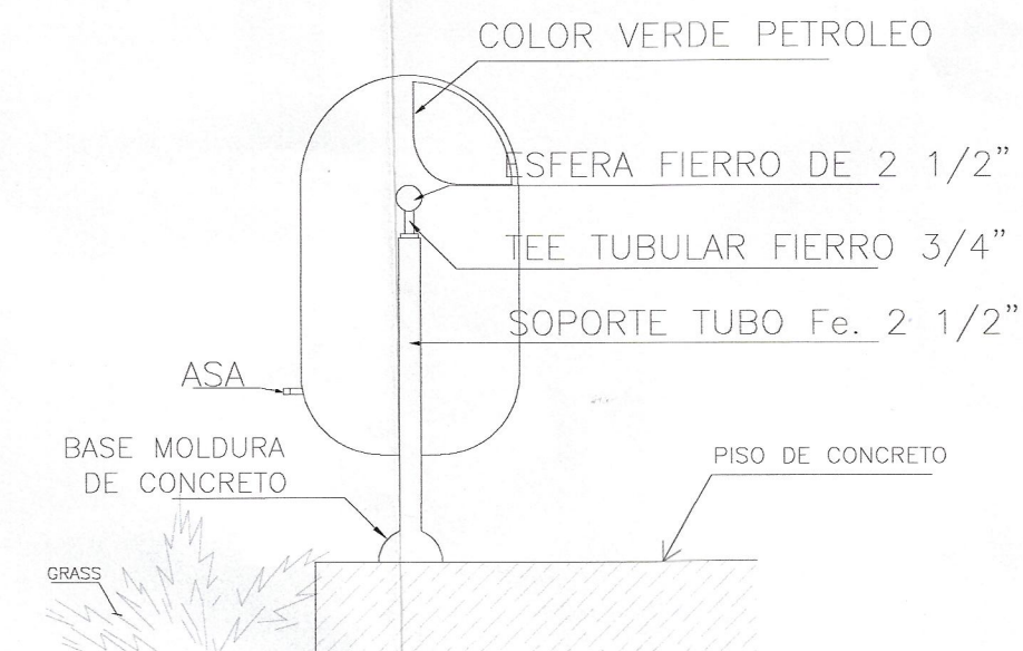
ELEVACION LATERAL TIPICA
