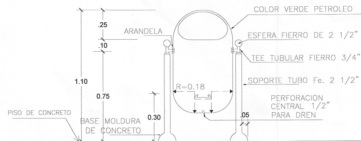
ELEVACION FRONTAL TIPICA
