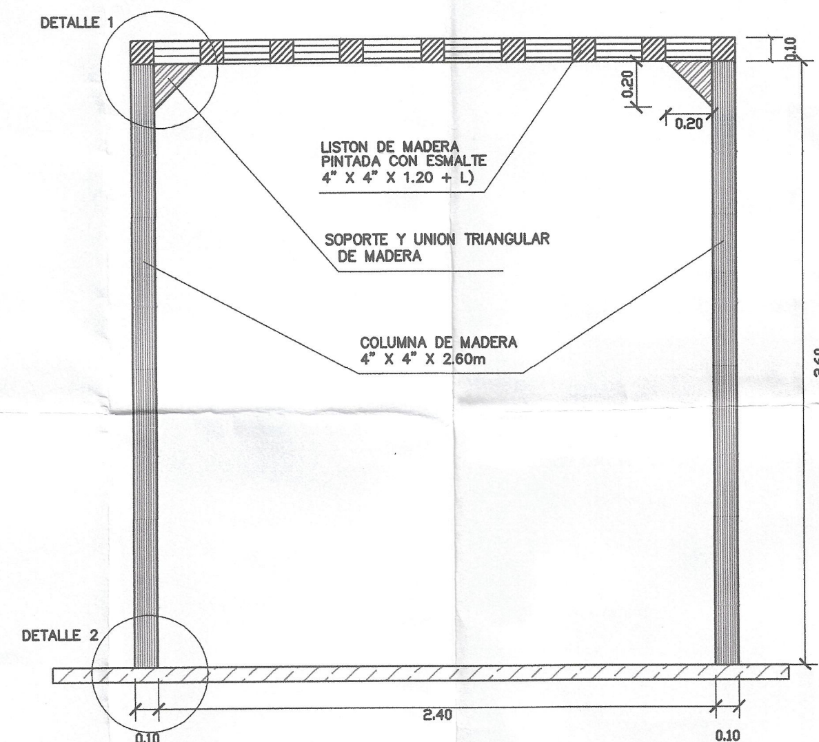
ELEVACION LATERAL (EL) PÉRGOLA DE MADERA ESC: 1/25
