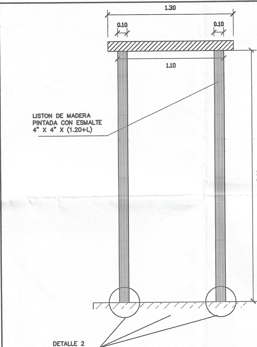
ELEVACION LATERAL (EL) PÉRGOLA DE MADERA ESC: 1/25
