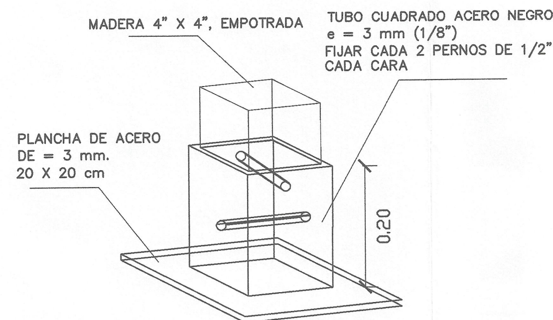
DETALLE 2 FIJACION Y EMBONE DE COMUNA EN BASE DE TERRAZO
