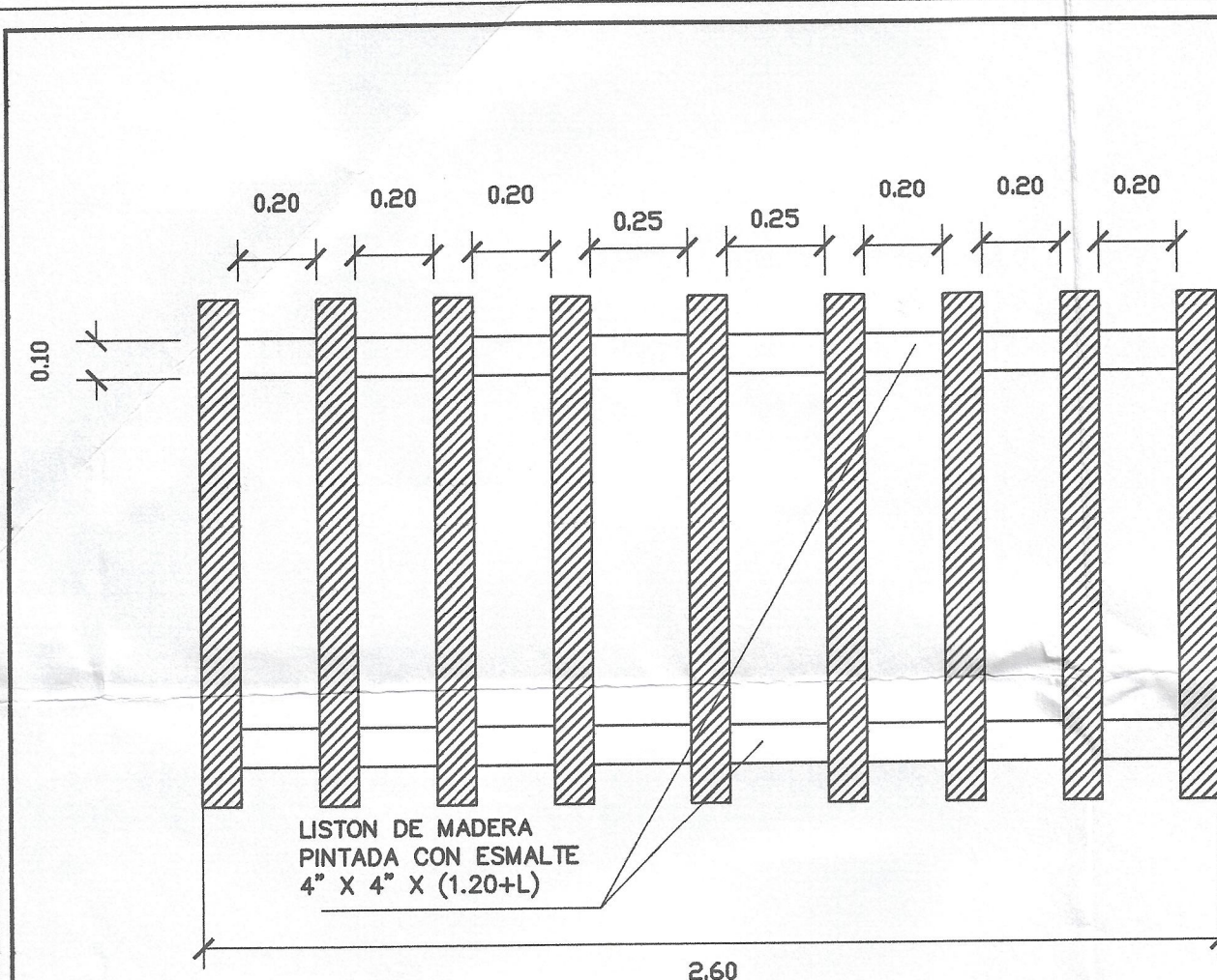
PLANTA PERGOLA DE MADERA
