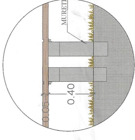
DETALLE DE MURETES ESC:1/20
