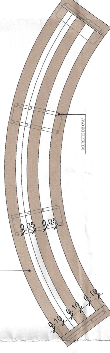
PLANO ESC:1/20
