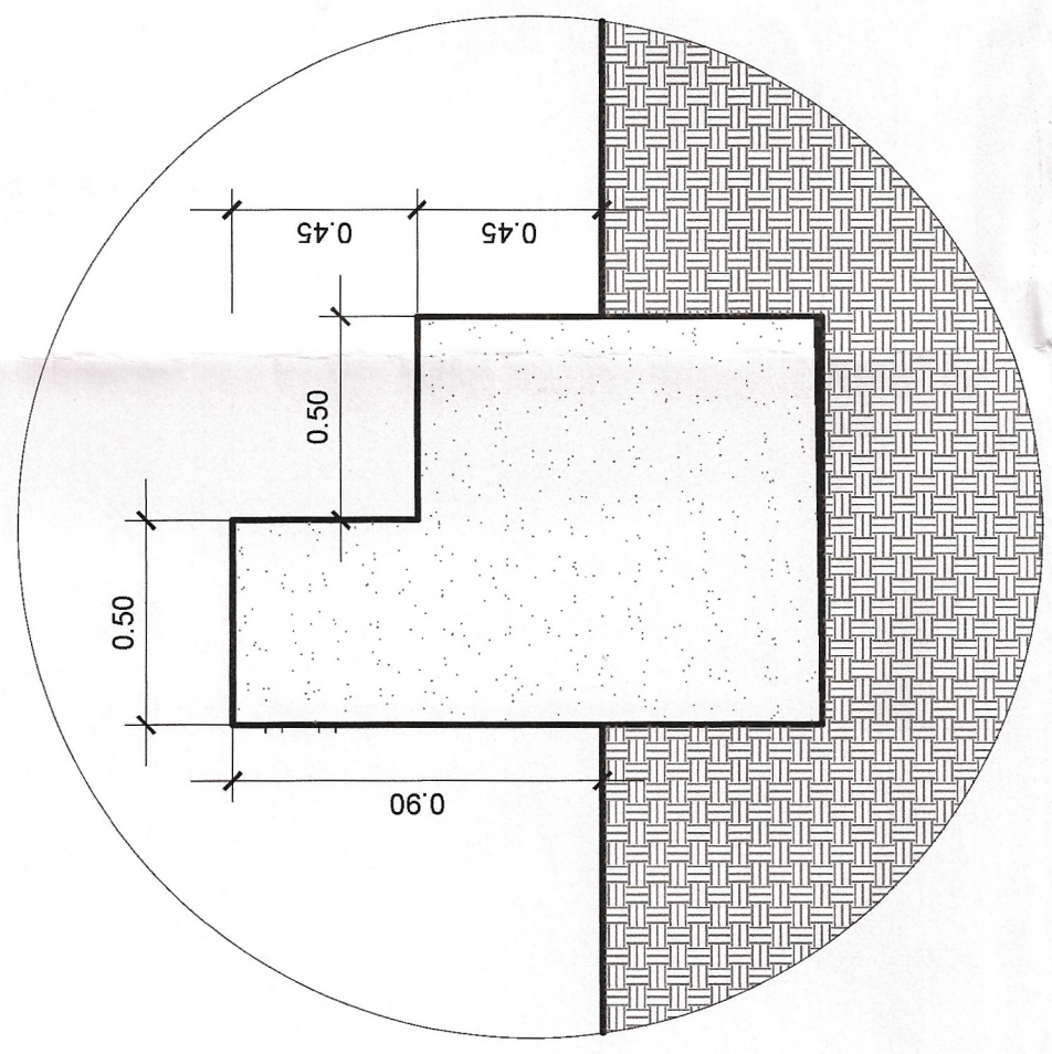
DETALLE DE GRADERIA
