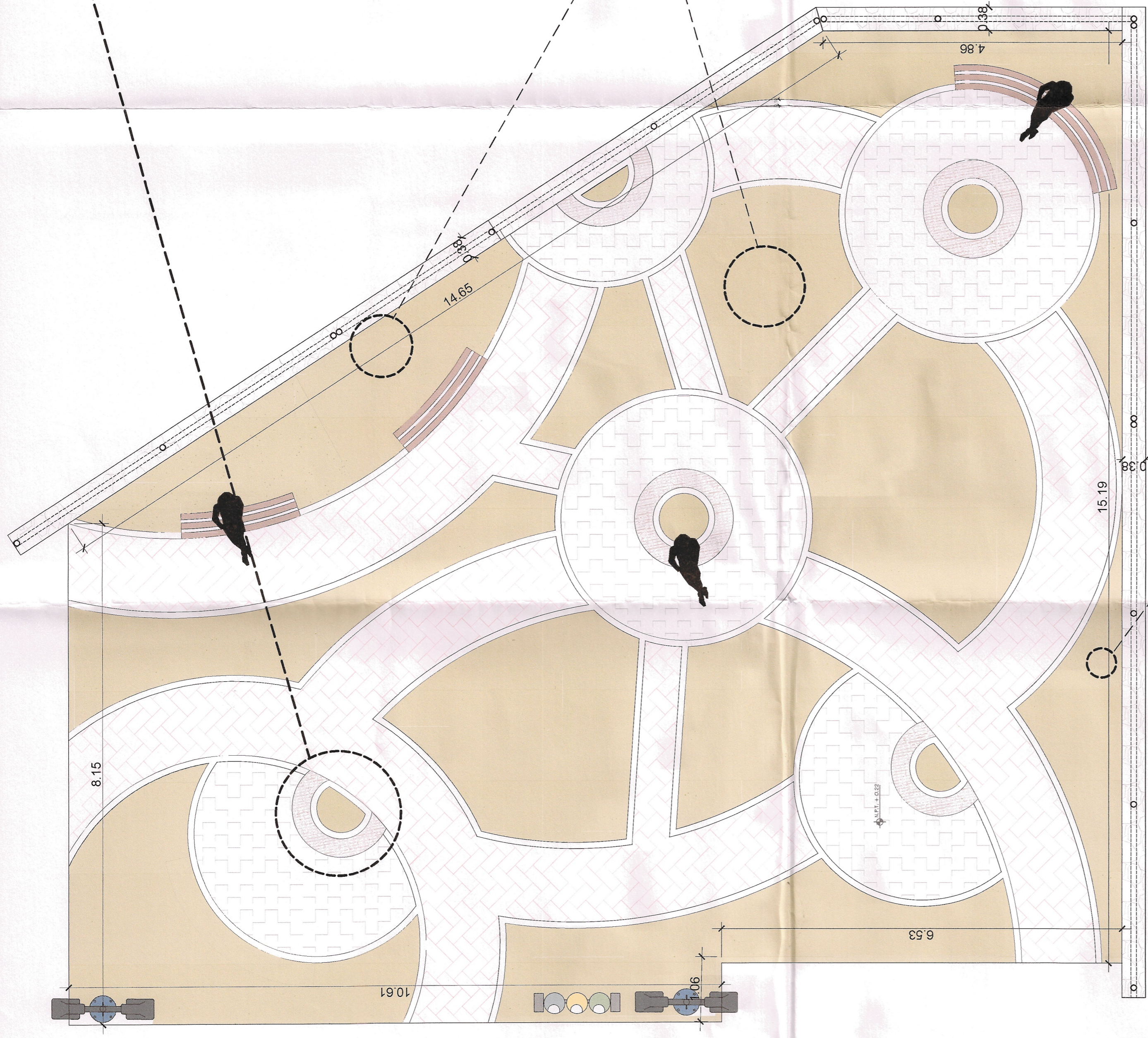
PLANO DE PROPUESTA ESC:1/50
