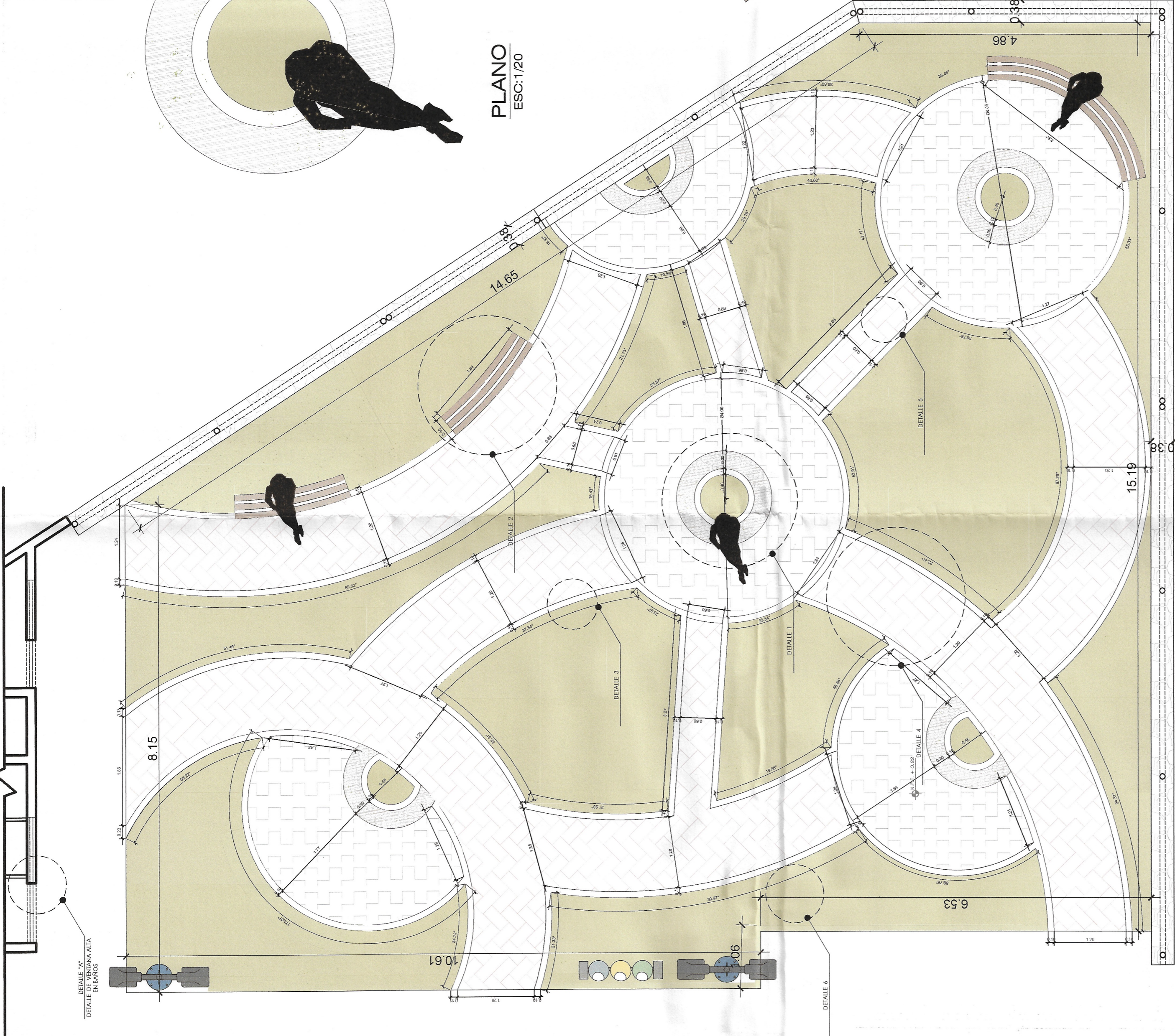
PLANO DE PROPUESTA ESC:1/50
