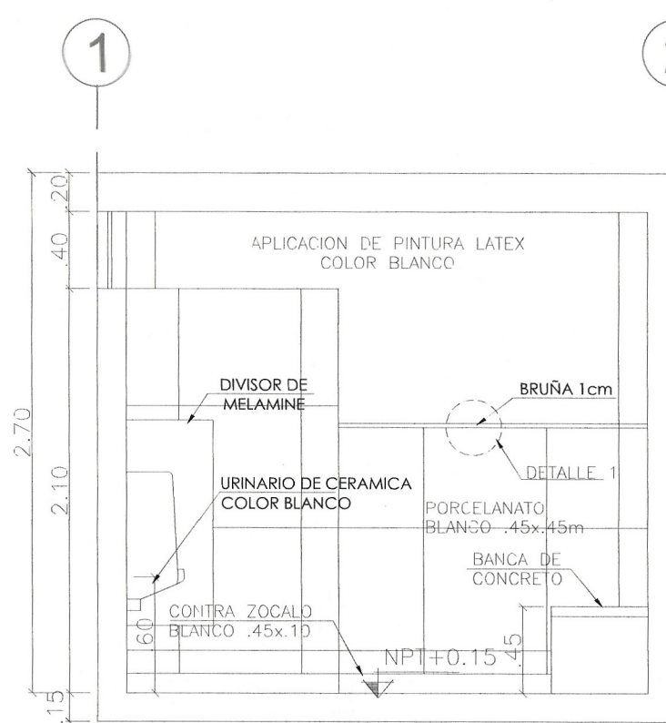
CORTE 4 esc 1:35
