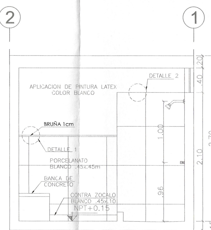
CORTE 5 esc 1:35
