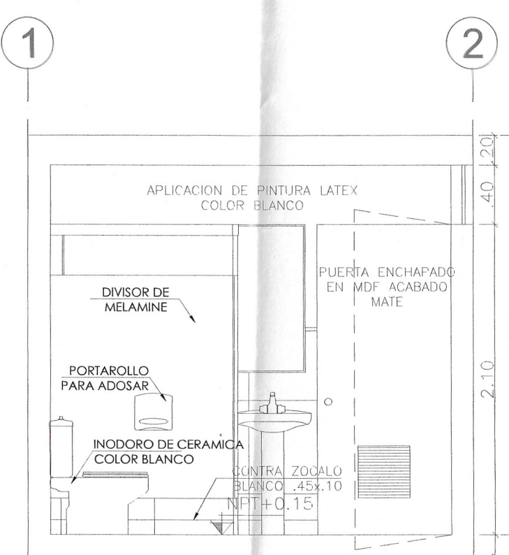
CORTE 6 esc 1:35
