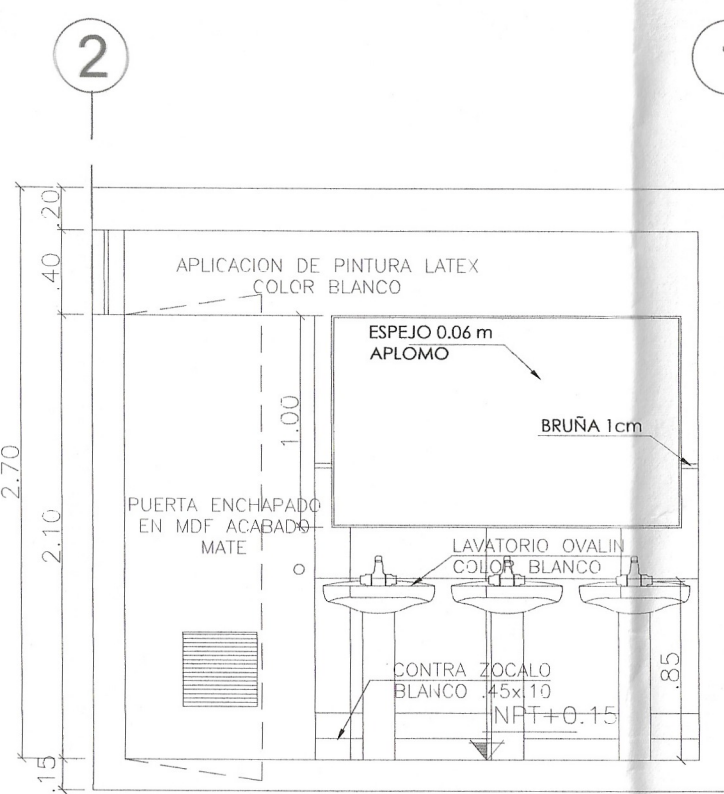
CORTE 3 esc 1:35
